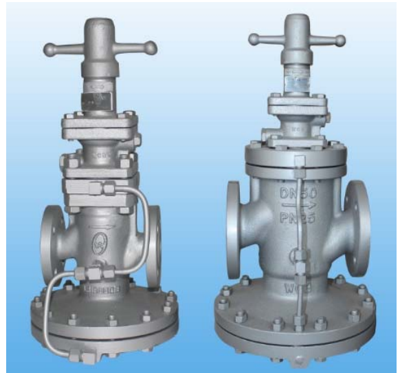
口径: DN15-25
