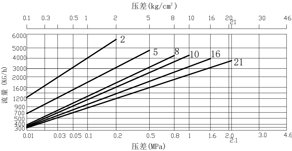
FFT45F / FFT45FU（DN40~DN50） 排量表
